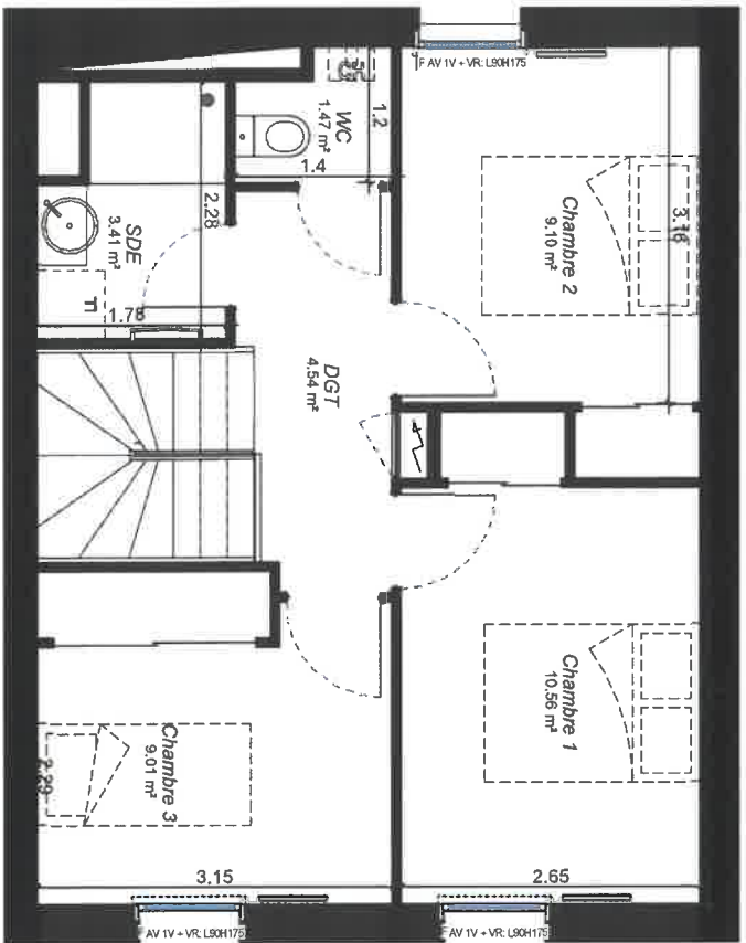
M01 R+1 1 : 50
