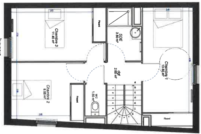
M.01 Plan R+0 1:30
