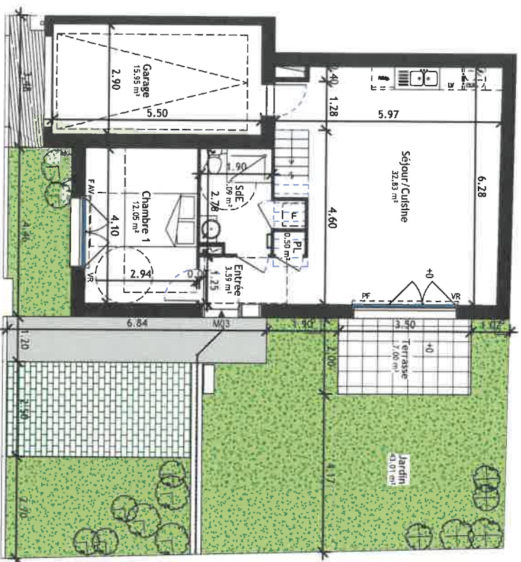
PDV - M03 - R+0 échelle = 1 : 100
