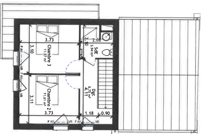
PDV - M03 - R+1 échelle = 1 : 100
