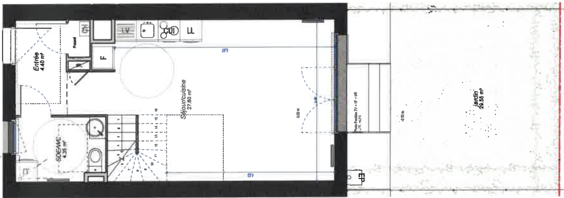
M.06 Plan BDC 1:50
