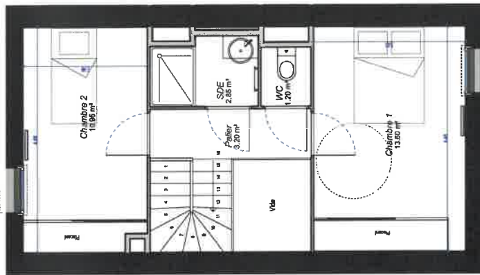
M.06 Plan R+1 1:50
