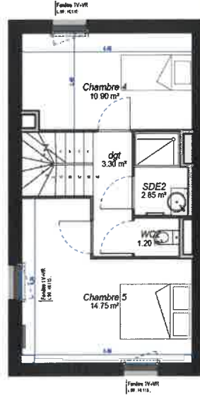
M.10 Plan R+2 1:80
