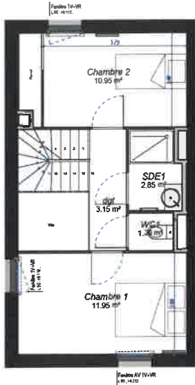
M.10 Plan R+1 1:80
