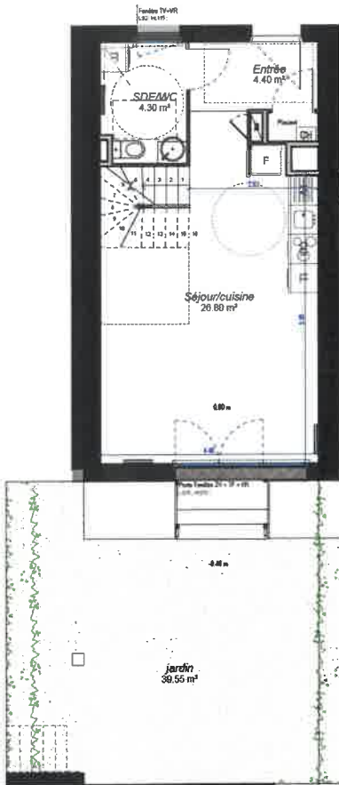
M.02 Plan RDC 1:88
