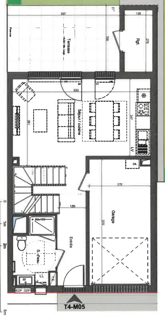
PLAN DE REZ-DE-CHAUSSEE
